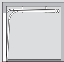
Prowadzenie Obniżone LH (sprężyny skrętne z tyłu)
