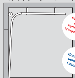
Prowadzenie Wysokie H (sprężyny skrętne z przodu)
