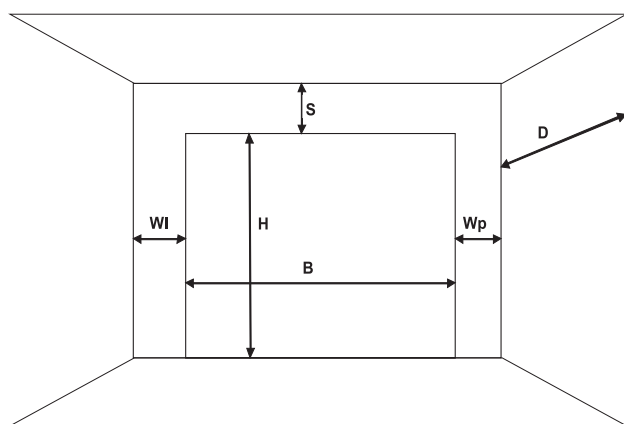
Bramy 40 mm - Prowadzenie STH i LH - Wymagania instalacyjne
