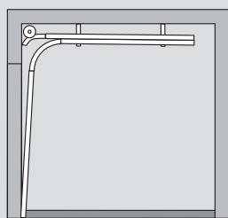
Prowadzenie Standardowe STH (sprężyny skrętne z przodu)
