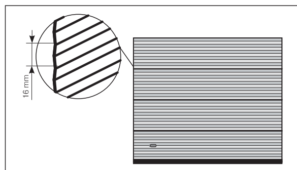
BRAMA STALOWA Z V-PROFILOWANIEM
