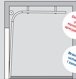
Nadproże Wysokie H (sprężyny skrętne z przodu)
